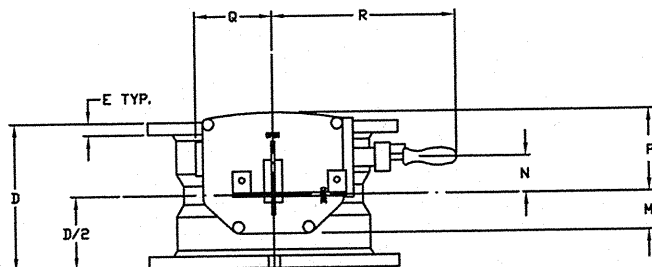
ACTUATOR POSITION 3
