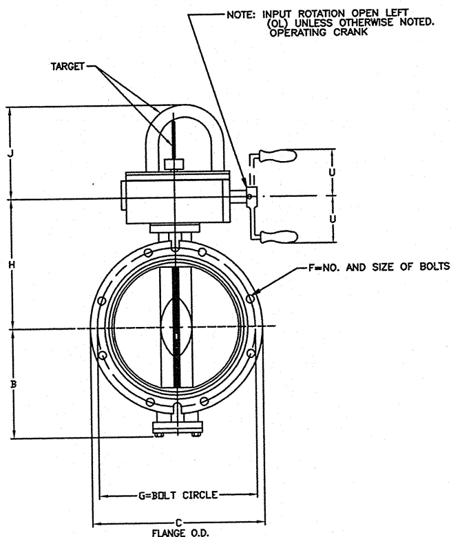
ACTUATOR POSITION 3
