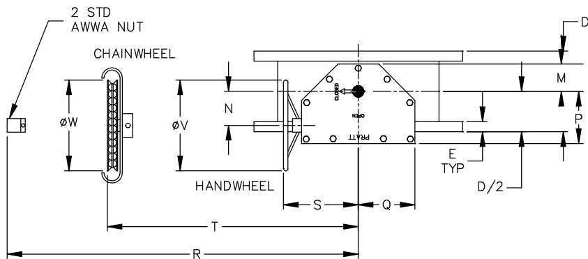
ACTUATOR POSITION 1
