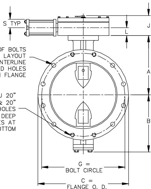
ACTUATOR POSITION 1
