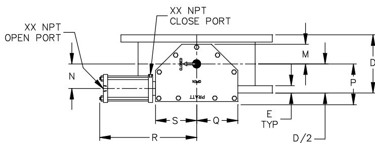
ACTUATOR POSITION 1
