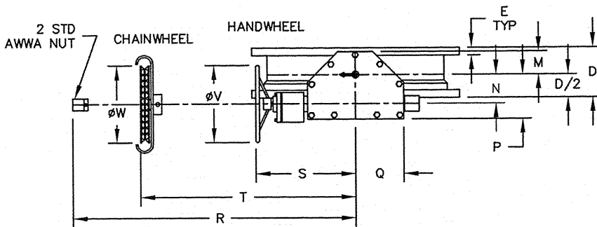
ACTUATOR POSITION 1
