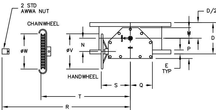
ACTUATOR POSITION 1
