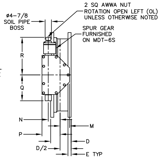
ACTUATOR POSITION 1
